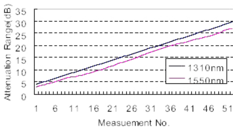
Variable Attenuator(Air-Gap:UPC-APC)
